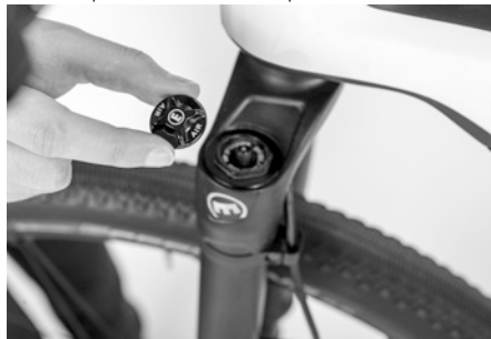
Fig. 43: Válvula de presión para ajustar la presión de la horquilla
