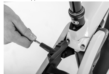
Fig. 41: Tornillos de sujeción/tija de sillín Dropper
