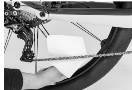
Fig. 21: Lubricar la cadena
