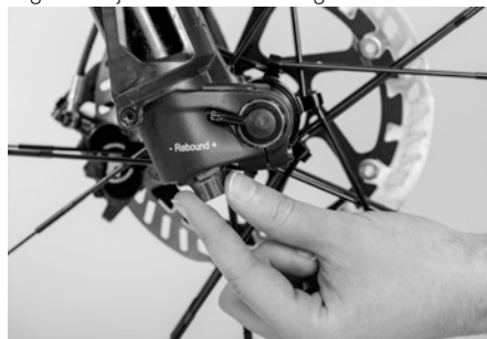
Fig. 44: Ajuste de la amortiguación
