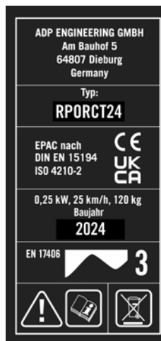
Fig. 1: Placa de características de ejemplo para PORSCHE EPAC
