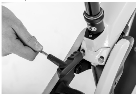
Fig. 41: Viti di bloccaggio / reggisella Dropper
