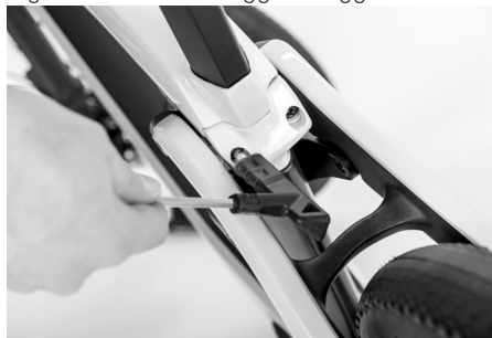
Fig. 40: Viti di bloccaggio / reggisella AERO
