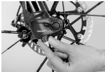
Abb. 44: Dämpfungseinstellung
